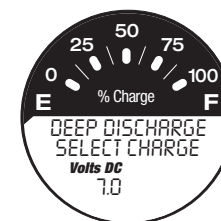
État de décharge profonde ; à partir de là il est possible d'effectuer un changement de sélection de réglage rapide (Quick Set Change Selection) correspondant à votre type de batterie.
