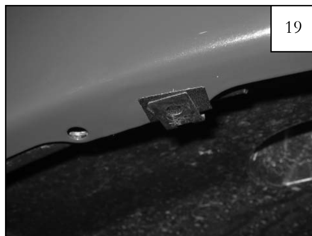
Install Clip (CL1-0022) over Tab (MT1-0014).
