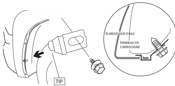
Levier Clip + Vis avec rondelle
