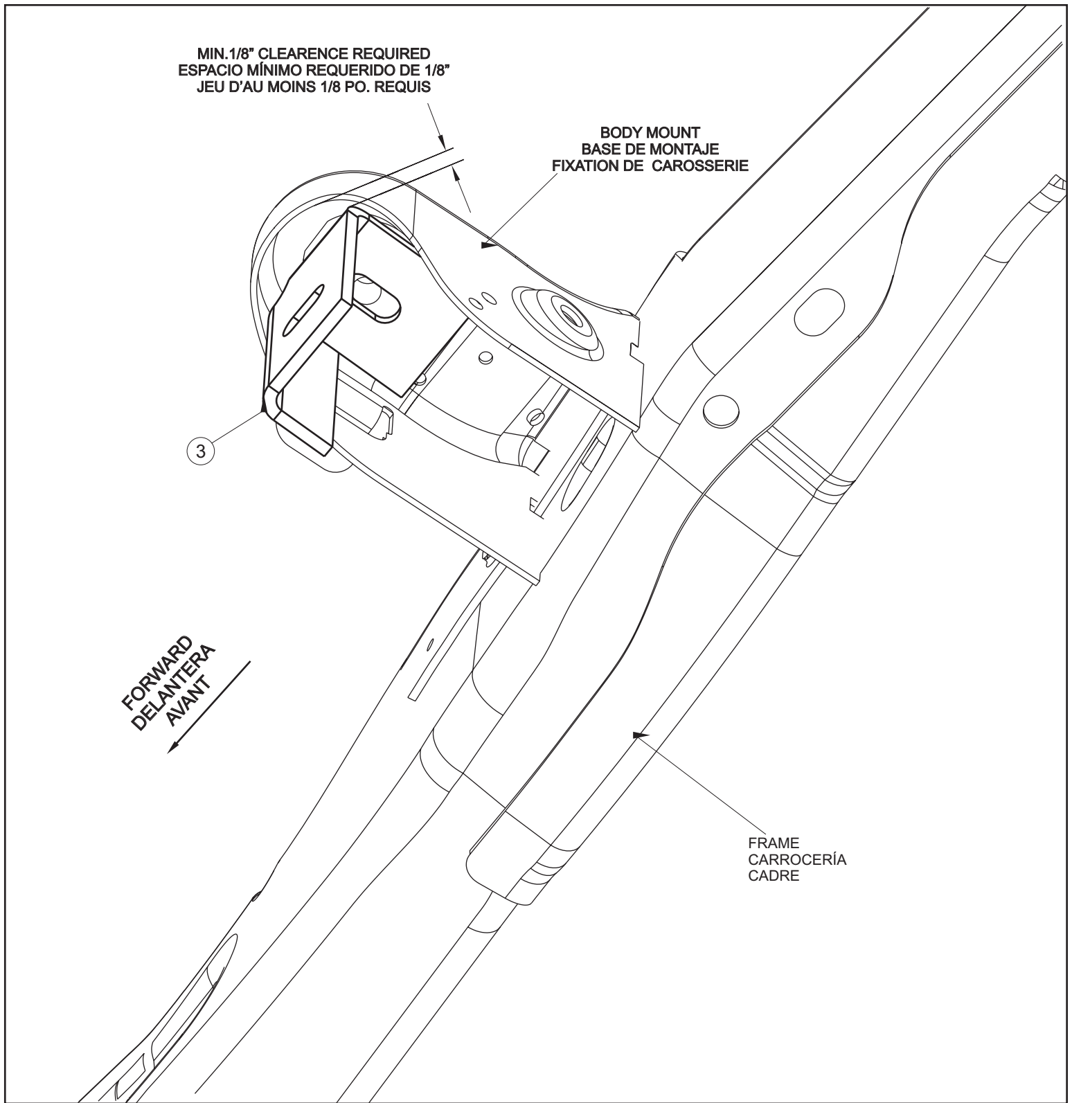
FIGURE 2 DRIVER SIDE FRONT BODY MOUNT FIGURA 2 BASE DE MONTAJE DELANTERA DEL LADO DEL CONDUCTOR FIGURE 2 FIXATION SUR LA CARROSSERIE, CÔTÉ CONDUCTEUR
