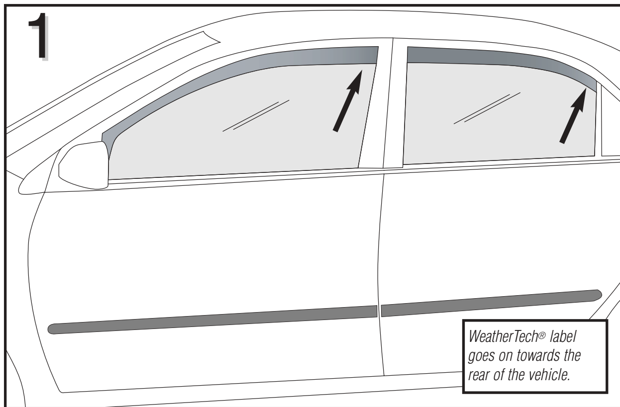
La etiqueta WeatherTech® va hacia la parte de atrás.
